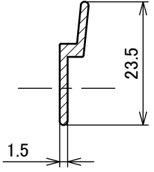
A部詳細図(S=1:1)
