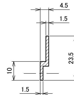
A部詳細図(S=1:1)
